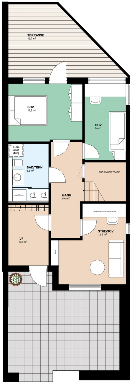
1. etasje
